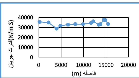
شکل ۹- روند تغییرات قدرت جریان در مقاطع مختلف Figure 9. The variation trend of flow power in different sections
