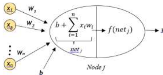
شکل ۳- ساختار یک نرون فرضی (تیفور (۴۴)) Figure 3. The structure of a hypothetical neuron (Tayfur (44))
