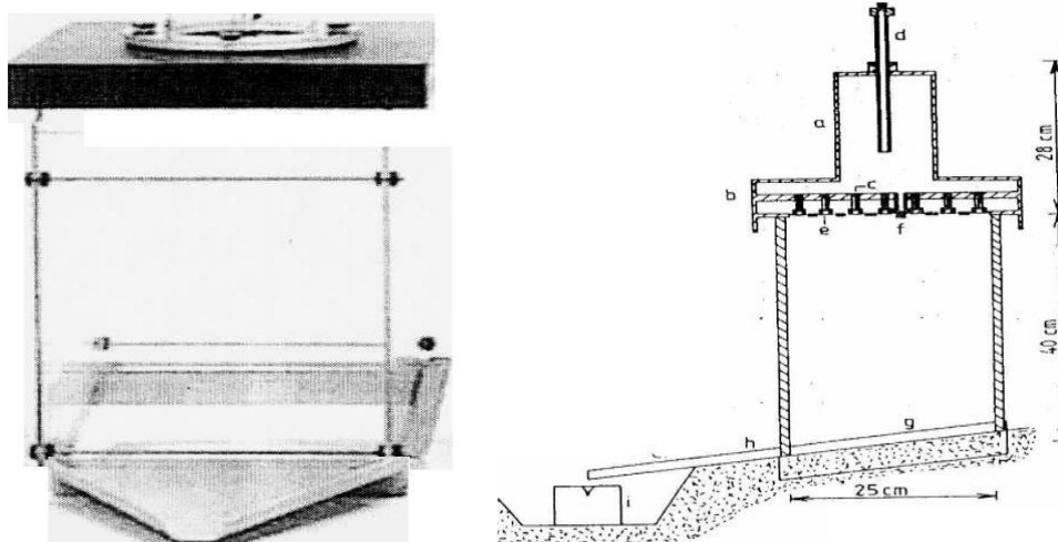
شکل ۲- نمایی کلی از شبیه‌ساز کامفورست در ارتفاع ۴۰ سانتی‌متری Figure 2. Total view of the kamphorst rain simulator in height 40 cm
