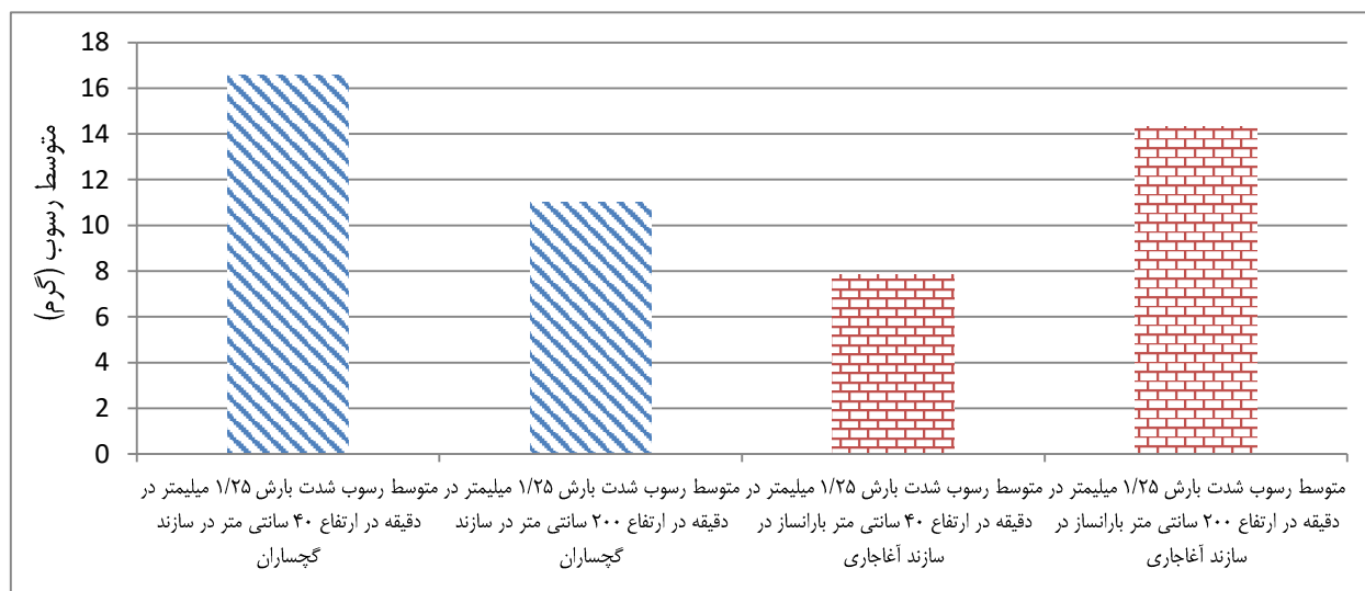
شکل ۵- مقایسه متوسط رسوب تولیدی در ارتفاع‌های مختلف شبیه‌ساز باران و در شدت ۱/۲۵ میلی‌متر در دقیقه در کاربری مرتع سازندهای گچساران و آگاهجاری
