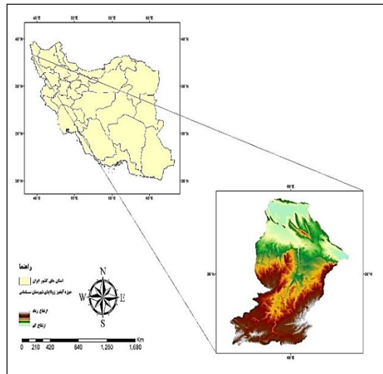
شکل ۱- موقعیت کشوری حوزه آبخیز زولاچای شهرستان سلماس (منبع: نگارندگان، ۱۳۹۸) Figure 1. Country location of Zolachai watershed in Salmas city
