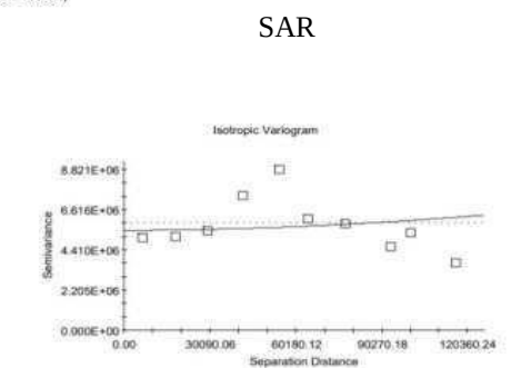
ادامه شکل ۶- واریوگرام‌های پارامترهای کیفی آب‌های زیرزمینی Continued Figure 6. Variograms of groundwater quality parameters
