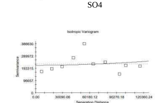
ادامه شکل ۶- واریوگرام‌های پارامترهای کیفی آب‌های زیرزمینی Continued Figure 6. Variograms of groundwater quality parameters
