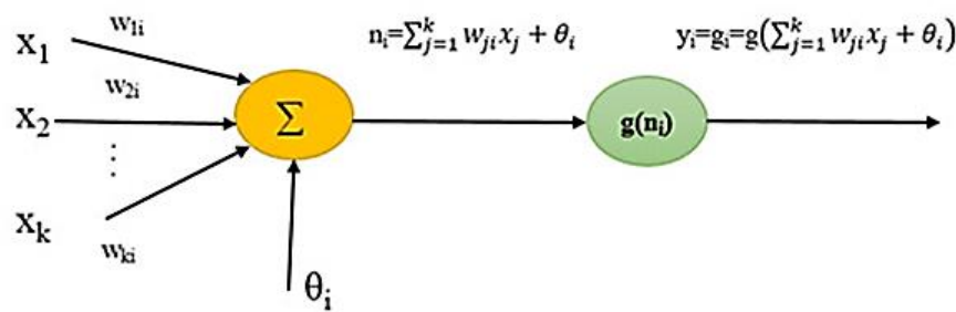
شکل ۳- یک نمونه از شبکه‌های عصبی مصنوعی
