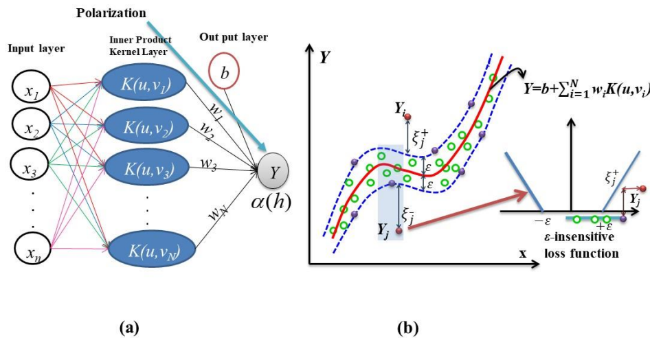
شکل ۴- نمونه‌ای از معماری ماشین بردار گرایی Figure 4. An example of regression vector machine architecture
