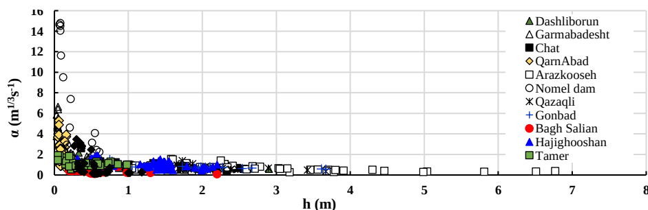
شکل ۶- تغییرات پارامتر \alpha نسبت به عمق جریان برای تمامی ایستگاه‌های هیدرومتری مورد مطالعه
