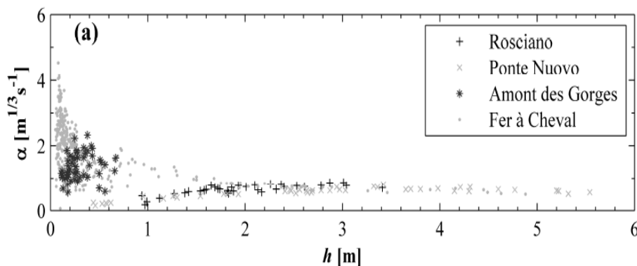
شکل ۲- منحنی \alpha - h برای چهار رودخانه مختلف در کشور ایتالیا (کوراتو و همکاران، ۲۰۱۴) Figure 2. \alpha - h Curves for four different rivers in Italy (Corato et al., 2014)
