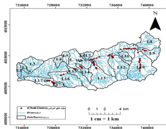
شکل ۲- زیرحوضه‌ها و بندهای اصلاحی حوزه آبخیز لنگر ۱ Figure 2. Sub-basins and chek dams of the Langar 1 watershed
