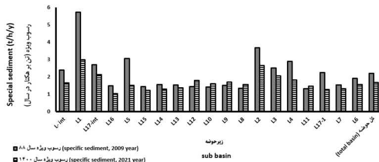
شکل ۳- ارزیابی رسوب ویژه حوزه آبخیز لنگر ۱
