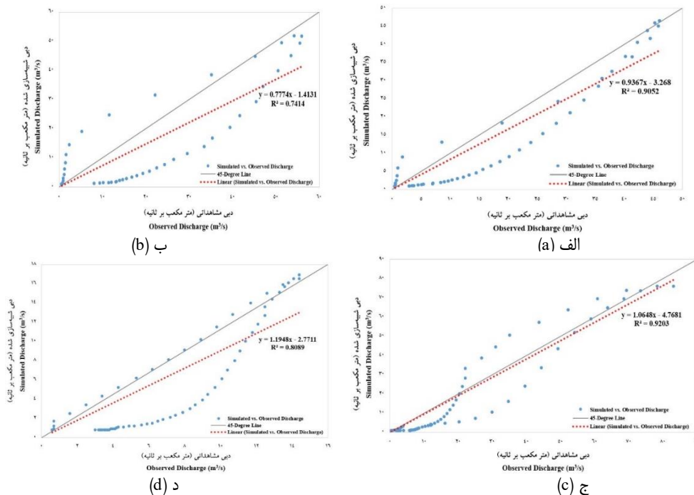
شکل ۵- نمودار پراکندگی دبی شبهه‌سازی شده و مشاهداتی (الف) ۱۳۹۰/۰۷/۱۲ (ب) ۱۳۹۰/۰۹/۲۰ (ج) ۱۳۹۴/۰۸/۲۳ (د) ۱۳۹۶/۰۹/۱۰ Figure 5. Scatter plots of Simulated and Observed Discharge a) 04 Oct. 2011 b) 11 Dec. 2011 c) 14 Nov. 2016 d) 01 Dec. 2017
