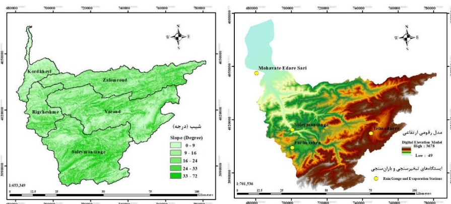
شکل ۱- نقشه مدل رقومی ارتفاعی و شیب حوزه آبخیز تاجن Figure 1. DEM and Slope Maps of the Tajan Watershed
