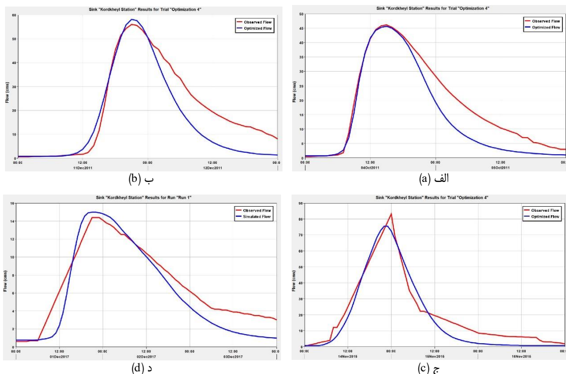
شکل ۳- هیدروگراف‌های مشاهداتی و محاسباتی (الف) ۱۳۹۰/۰۷/۱۲ (ب) ۱۳۹۰/۰۹/۲۰ (ج) ۱۳۹۴/۰۸/۲۳ (د) ۱۳۹۶/۰۹/۱۰ Figure 3. Observed and Calculated Hydrographs a) 04Oct.2011 b) 11Dec.2011 c) 14Nov.2016 d) 01Dec.2017
