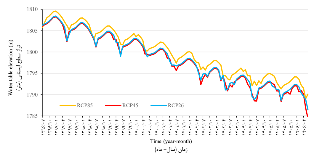
شکل ۵- هیدروگراف آبخوان در طول دوره پیش‌بینی تحت سناریوهای RCP2.6، RCP4.5 و RCP8.5 Figure 5. Aquifer hydrographs during forecast period under the RCP2.6, RCP4.5, and RCP8.5 scenarios
