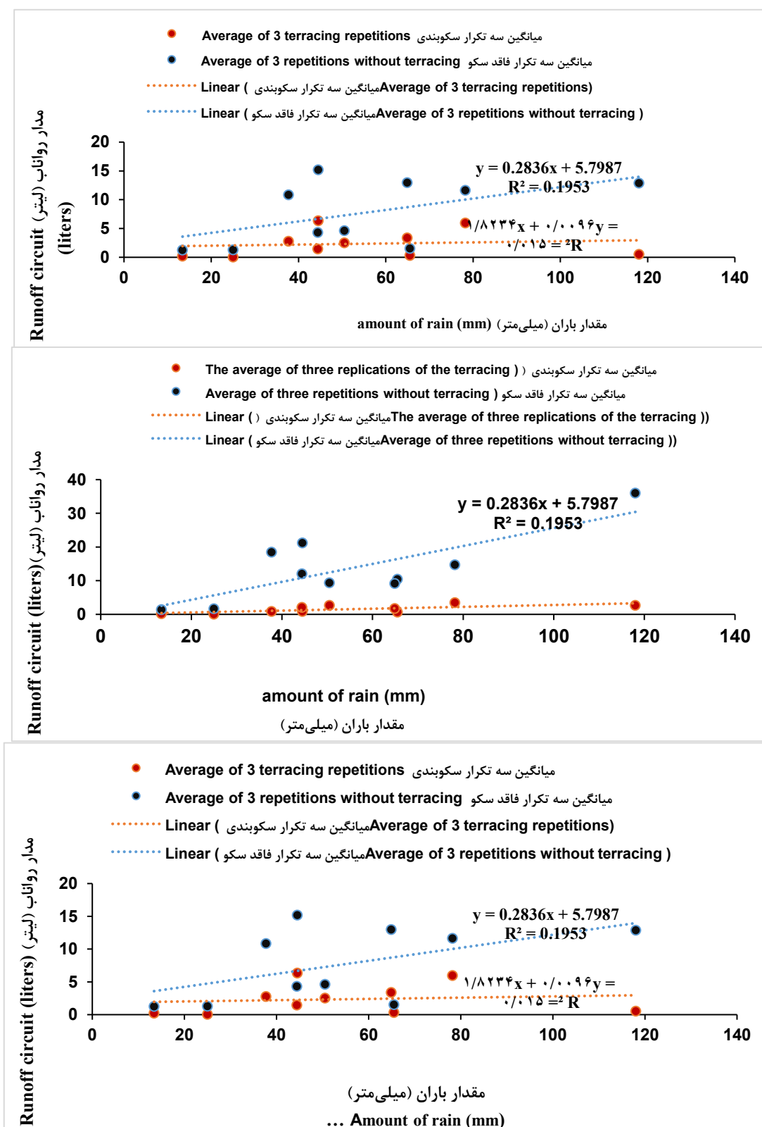
شکل ۴- رابطه همبستگی بین مقدار بارش و حجم رواناب در اراضی سکوبندی و فاقد سکوبندی در سایت‌های اول (بالا)، دوم (وسط) و سوم (پایین)
