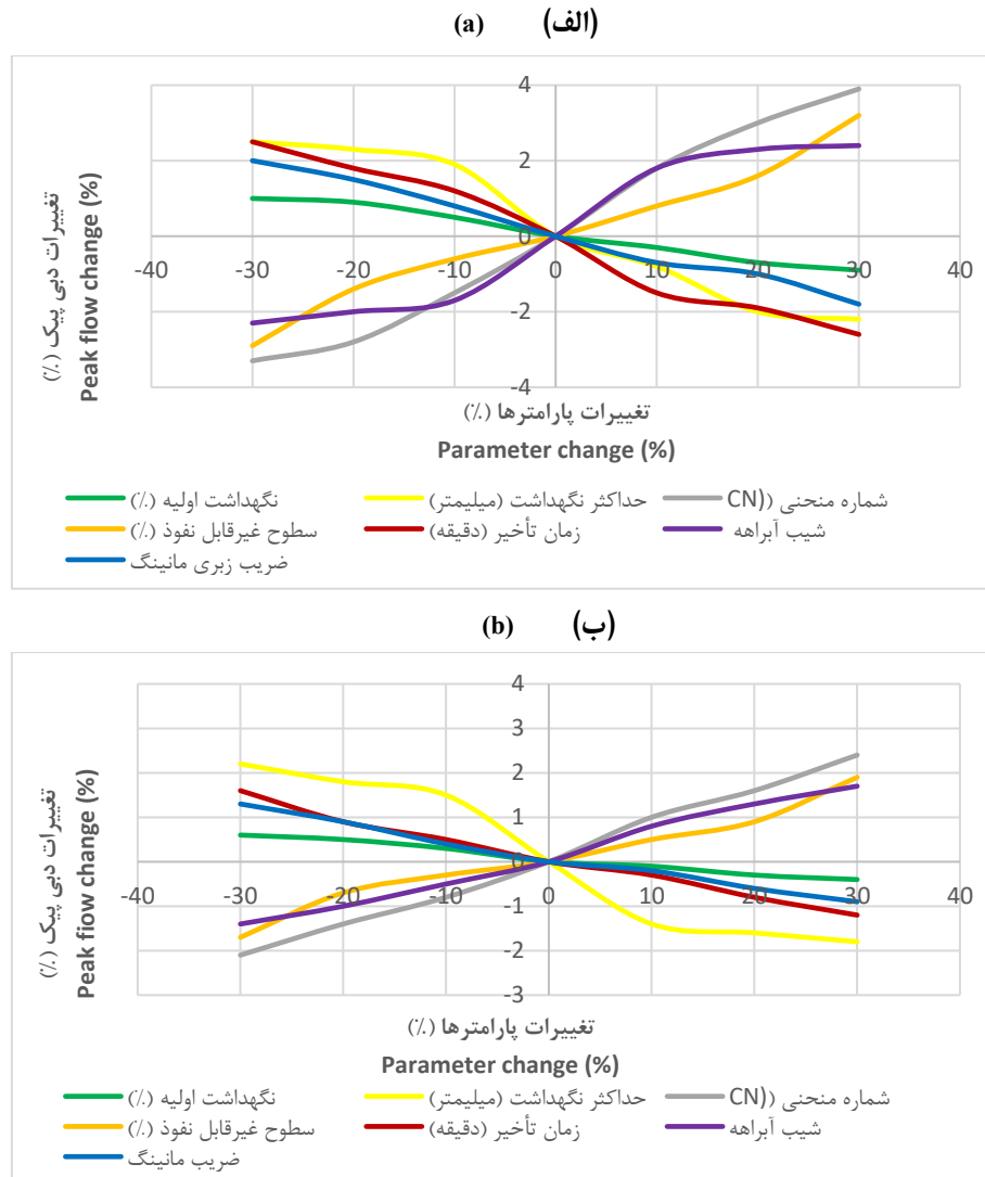
شکل ۸- حساسیت تغییرات پارامترها نسبت به دبی اوج رواناب برای (الف): حوضه شاهد و (ب): حوضه احیا شده Figure 8. The sensitivity of parameter changes to peak runoff flow for (a): control and (b): restored watersheds
