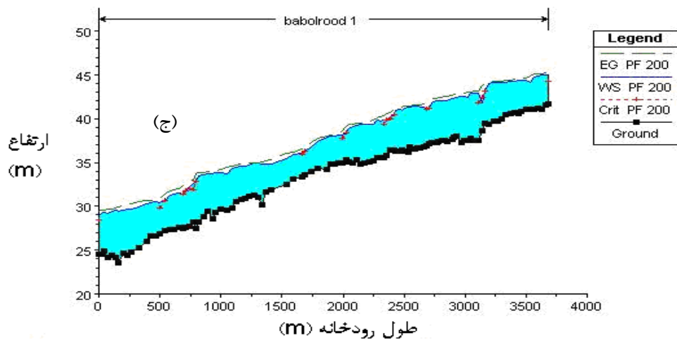
شکل ۲- نیمرخ های طولی سطح آب برای بازه ۴۰۰۰ متری در رودخانه بابلرود برای دوره‌های بازگشت: الف) ۲ سال، ب) ۲۵ سال و ج) ۲۰۰ سال.
