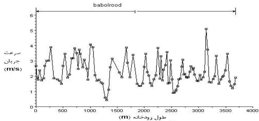
شکل ۳- الف) تغییرات عمق بیشینه (m) جریان سیلاب و ب) تغییرات سرعت ( ms^{-1} ) جریان سیلاب، برای دوره بازگشت ۲۵ ساله در بازه ۴۰۰۰ متری مورد بررسی در رودخانه بابلرود.
