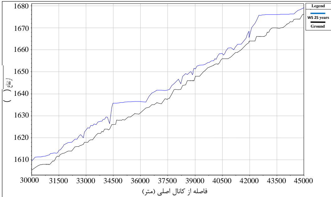
شکل ۵- شبیه سازی پروفیل طولی در شرایط طبیعی برای زیر بازه ۱ به ازای سیلاب با دوره بازگشت ۲۵ سال
