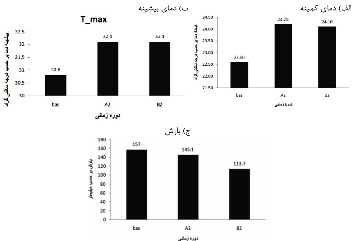
شکل ۶- مقایسه دمای بیشینه، دمای کمینه و بارش ایستگاه سینوپتیک جاسک در دوره پایه و دوره آتی تحت سناریوی‌های A2 و B2
