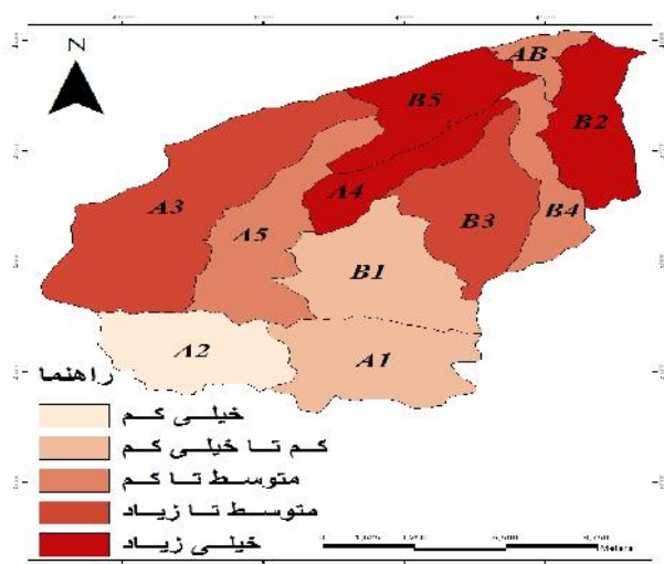
شکل ۴- اولویت بندی زیرحوزه‌ها بر اساس پارامترهای مورفومتری
