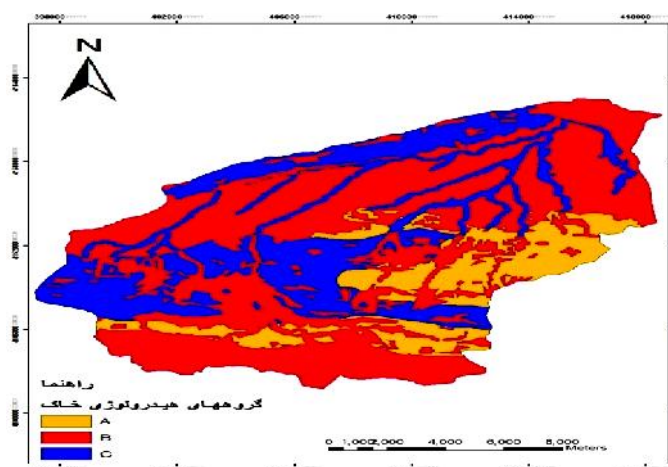
شکل ۶- گروه‌های هیدرولوژیکی خاک حوزه آبخیز لهنذر
