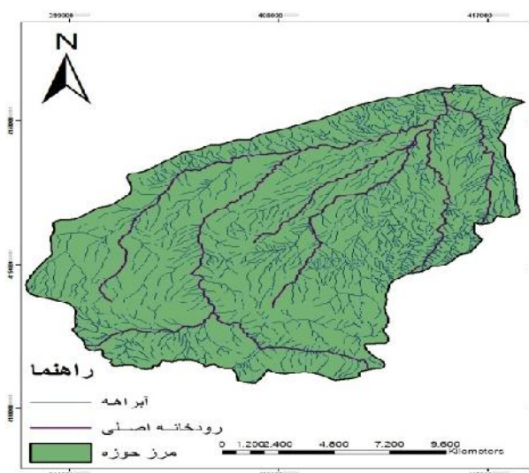
شکل ۳- شبکه آبراه‌ای و زهکشی حوزه لهن‌در
