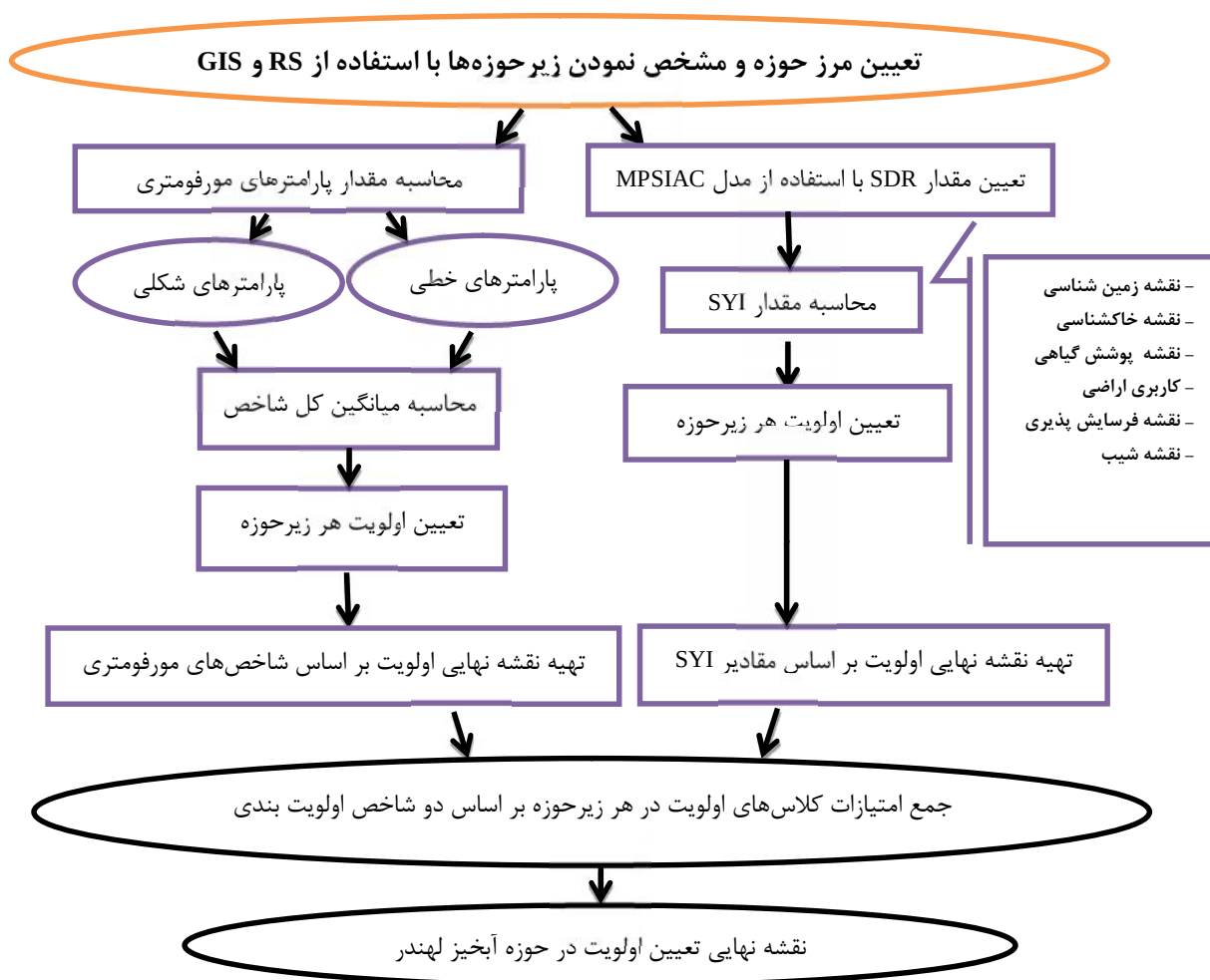
شکل ۲- نمودار روند تهیه نقشه نهایی اولویت زیر حوزه‌ها
