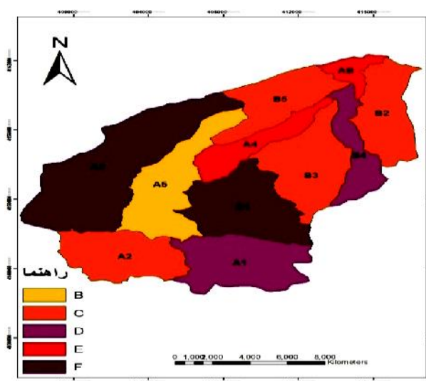
شکل ۷- اولویت‌بندی زیرحوزه‌های آبخیز لهندر بر اساس شاخص SYI
