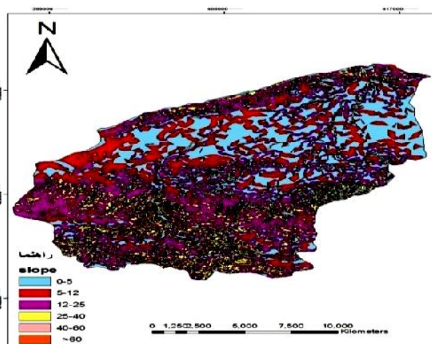
شکل ۵- طبقه‌بندی مقادیر شیب حوزه لهنذر
