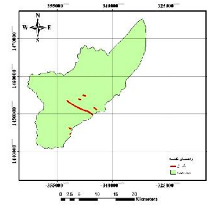
شکل ۶- نقشه پراکنش گسل در حوزه آبخیز شلمانرود
