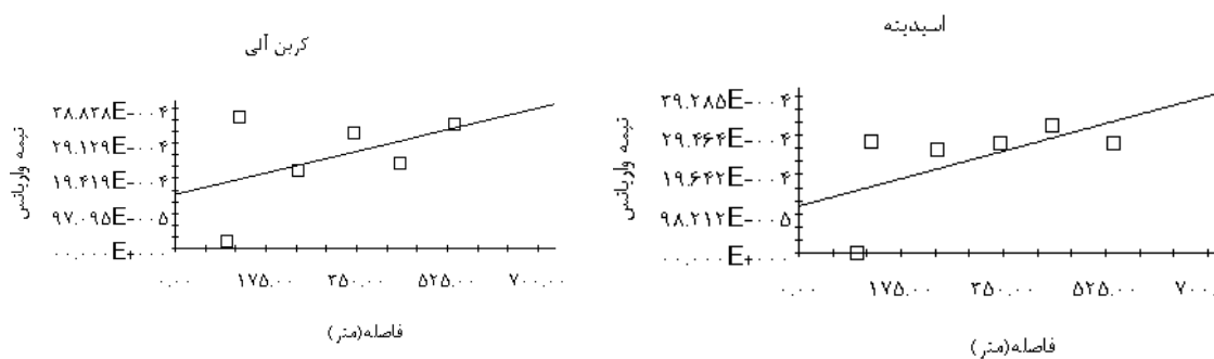
شکل ۲- مدل‌های واریوگرام برخی از خصوصیات خاک در منطقه کلید
