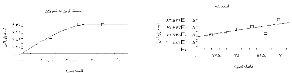
شکل ۴- مدل های واریوگرام برخی از خصوصیات خاک در منطقه بحرانی
