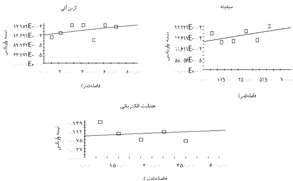
شکل ۳- مدل های واریوگرام برخی از خصوصیات خاک در منطقه مرجع
