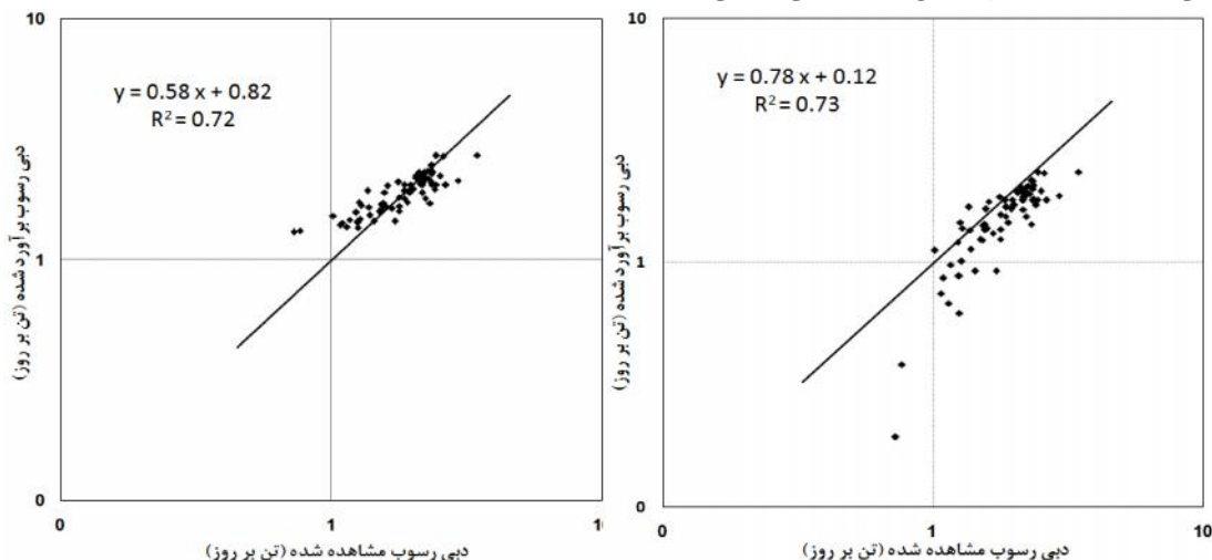
شکل ۳- نمودار پراکندگی داده‌های مشاهده شده و برآورد شده به روش منحنی سنجه (سمت راست) و ANFIS (سمت چپ)
