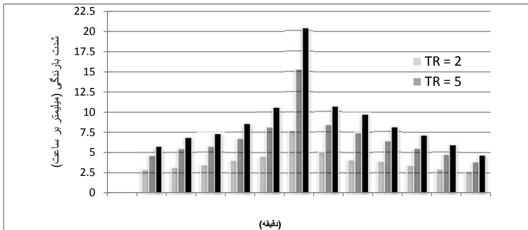
شکل ۲- هایتوگراف بارندگی ۲ ساعته برای دوره بازگشت‌های ۲، ۵ و ۱۰ ساله
