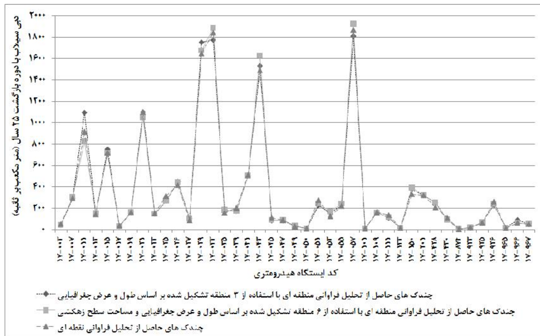
شکل ۳- برآورد سیلاب با دوره بازگشت ۲۵ سال با استفاده از تحلیل فراوانی منطقه‌ای و نقطه‌ای در حوزه‌ی سفیدرود
