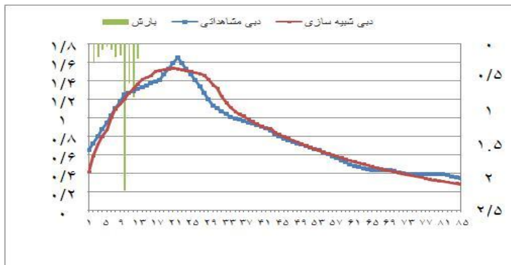
شکل ۴- هیدروگراف شبیه سازی و مشاهداتی در مرحله اعتبارسنجی
