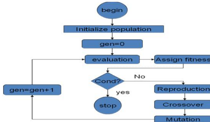
شکل ۳- فلوچارت الگوریتم ژنتیک (وب سایت ویکیپدیا)
