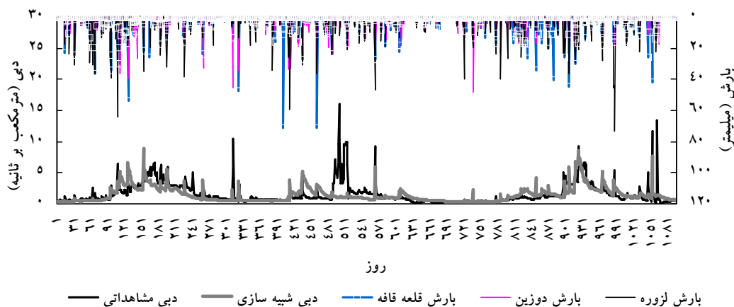
شکل ۶- نمودار روزانه دبی مشاهداتی و شبیه‌سازی شده دوره سه ساله (۸۶ - ۱۳۸۳) اعتبارسنجی حوزه آبخیز چهل‌چای
