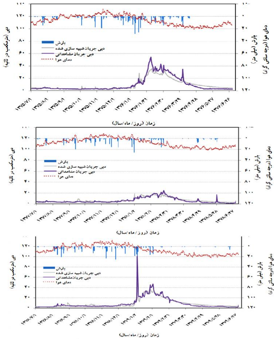
شکل ۵- مقایسه هیدروگراف روزانه شبهه‌سازی شده و مشاهده‌ای حوزه آبخیز طالقان در دوره واسنجی
