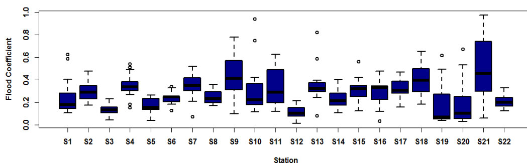
شکل ۴- نمودار جعبه‌ای تغییرات ضریب سیلابی طی دوره‌های مطالعاتی در ۲۲ ایستگاه هیدرومتری منتخب در استان اردبیل Figure 4. Box plot of flood coefficient variability during the study periods in 22 selected hydrometric stations of Ardabil province
