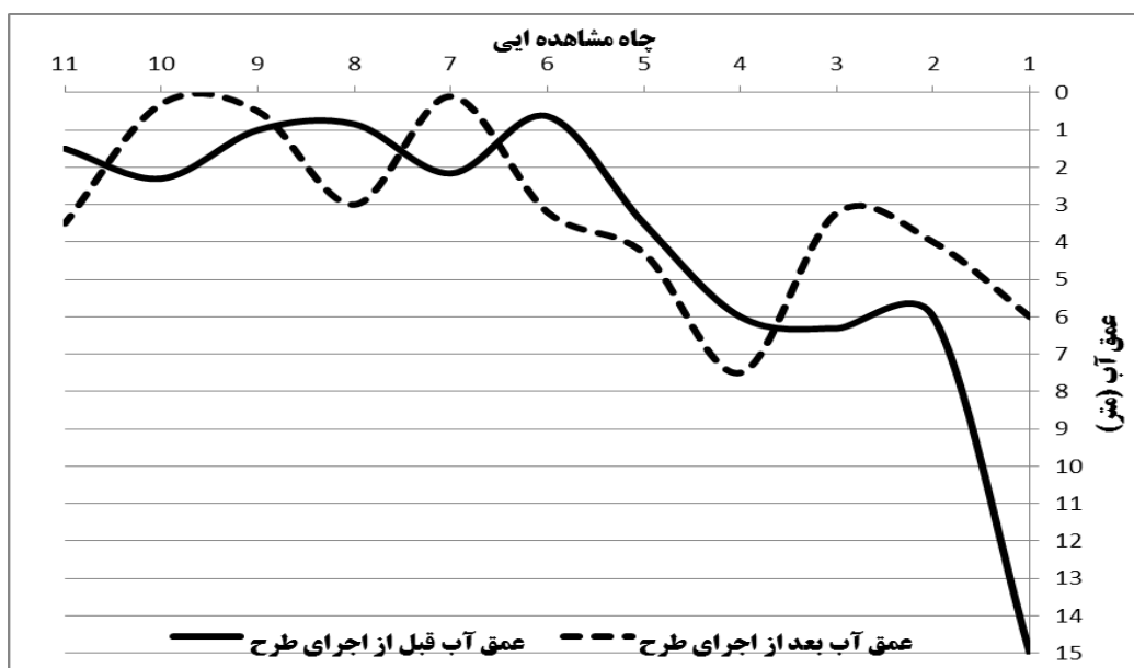
شکل ۸- مقایسه عمق آب قبل و بعد از اجرای طرح شبکه آبیاری و زهکشی البرز در شرایط بهینه برداشت از آب زیرزمینی
