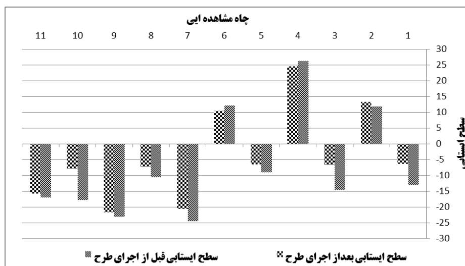
شکل ۶- مقایسه سطح ایستابی قبل و بعد از اجرای شبکه آبیاری و زهکشی البرز Figure 6. Compare of water heads before and after Alborz Irrigation and Drainage Network Performance
