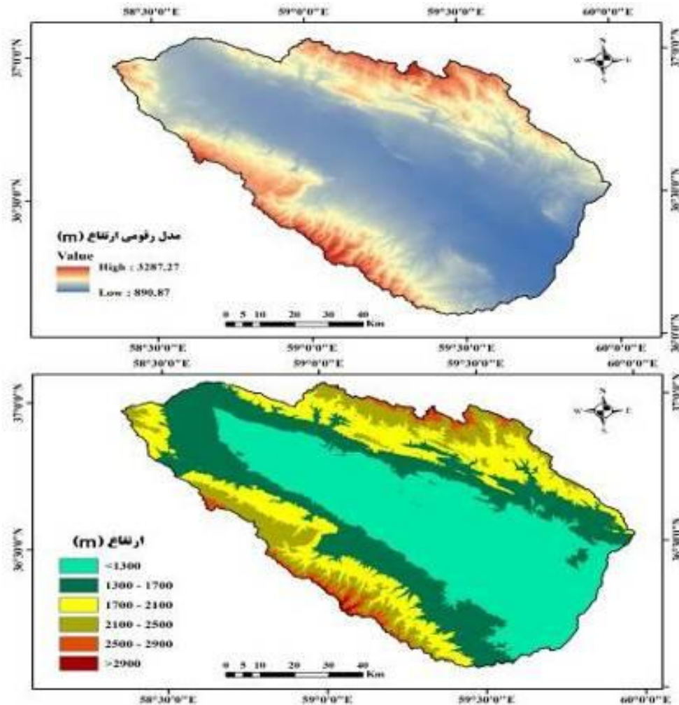
شکل ۲- نقشه‌های مدل رقمی ارتفاع (DEM) حوزه Figure 2. Maps of Digital Elevation Model (DEM) the watershed
