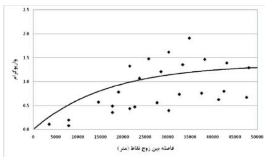
شکل ۲- نیم تغییرنمای تجربی و تئوری برای آبخوان آستانه-کوچصفهان Figure 2. The Empirical and Theory Semi-Variogram for Astane-koochesfahan Aquifer
