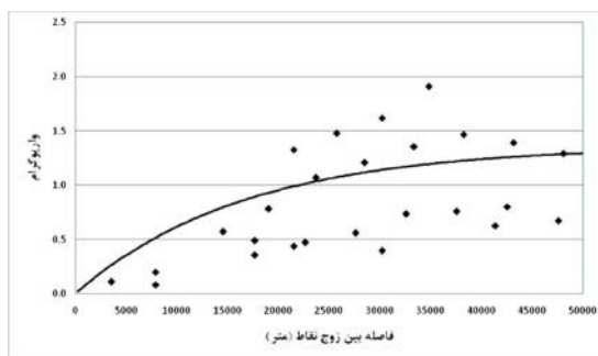
شکل ۲- نیم‌تغییرنمای تجربی و تئوری برای آستانه-کوچصفهان Figure 2. The Empirical and Theory Semi-Variogram for Astane-koochesfahan Aquifer
