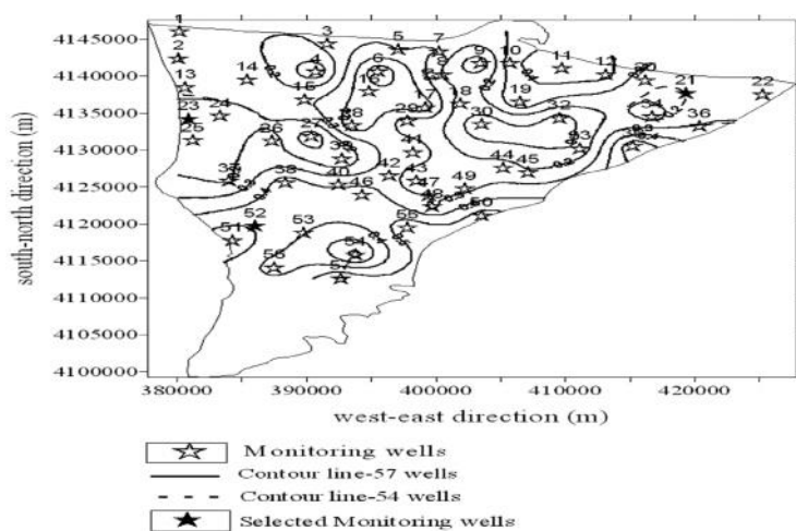
شکل ۴- منحنی‌های تراز سطح ایستابی با حذف سه چاه مشاهده‌ای به وسیله‌ی الگوریتم ژنتیک
