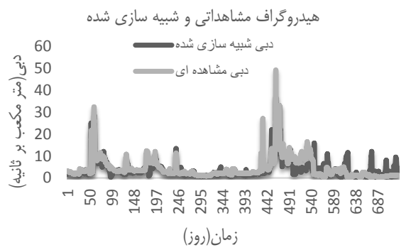
شکل ۱۱- هیدروگراف مشاهده‌ای و شبیه‌سازی شده برای دوره اعتبارسنجی (مقیاس ماهانه، ۱۳۸۷-۱۳۸۹) Figure 11. Observed and simulated hydrograph of validation (Monthly scale,1387-1389)
