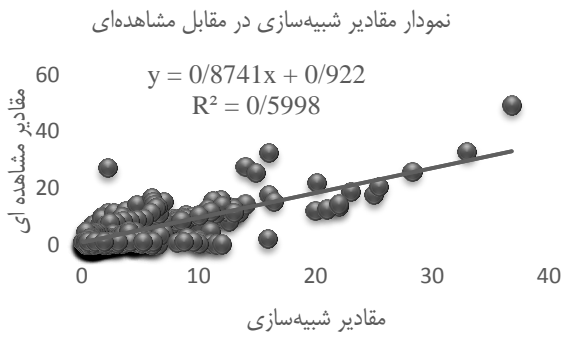
شکل ۱۲- مقایسه دبی متوسط ماهانه مشاهده‌ای و محاسباتی برای دوره اعتبارسنجی (مقیاس ماهانه، ۱۳۸۷-۱۳۸۹) Figure 12. Compare observed and simulated average monthly flow of validation (monthly scale, 1387-1389)
