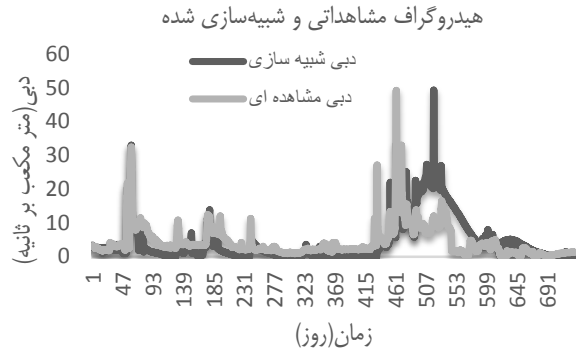
شکل ۹- هیدروگراف مشاهده‌ای و شبیه‌سازی شده برای دوره اعتبارسنجی (مقیاس روزانه، ۱۳۸۷-۱۳۸۹) Figure 9. Observed and simulated hydrograph of validation (Daily scale,1387-1389)
