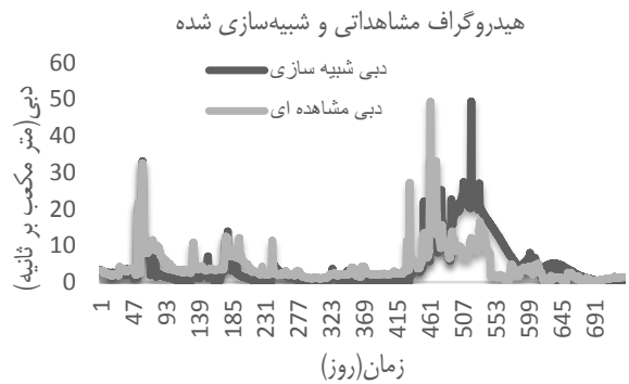
شکل ۱۳- هیدروگراف مشاهده‌ای و شبیه‌سازی شده برای دوره اعتبارسنجی (مقیاس سالانه، ۱۳۸۷-۱۳۸۹) Figure 13. Observed and simulated hydrograph of validation (Annual scale,1387-1389)
