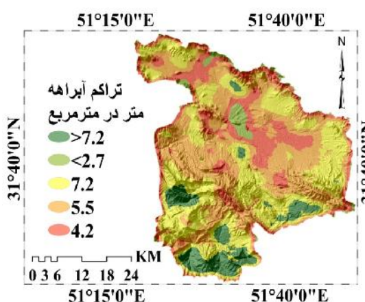
شکل ۷- نقشه تراکم آبراهه Figure 7. stream density map
