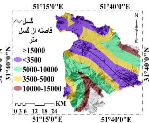
شکل ۱۰- فاصله از گسل Figure 10. Distance from fault
