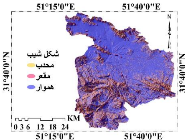
شکل ۶- نقشه شکل شیب Figure 6. Plan curvature map index
