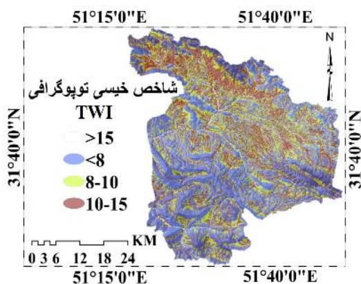
شکل ۵- نقشه شاخص رطوبت Figure 5. Topography wetness
