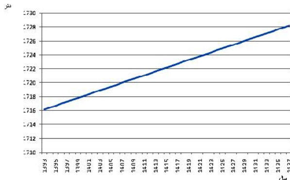
شکل ۳- مسیر بهینه ارتفاع سطح سفره آب زیرزمینی در دشت همدان- بهار Figure 3. Optimal path of altitude groundwater in the plain of Hammedan - Bahar
