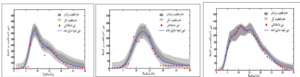
شکل ۴- تخمین عدم قطعیت کل (ناحیه رنگ روشن)، عدم قطعیت پارامتر (ناحیه رنگ تیره)، جریان مشاهده‌ای (نقاط دایره‌ای) و آبنمود بهترین شبیه سازی (خط تیره) Figure 4. Total prediction uncertainty bounds (lighter shaded region), the uncertainty bounds of parameter (darker shaded region), observed stream flows (dots), best simulation (solid line)
