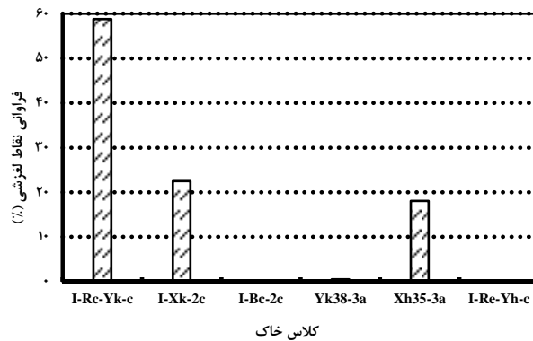
شکل ۴- نمودار درصد فراوانی نقاط لغزشی در هر کلاس خاک Figure 4. Plot offfrequency percentage of landslide points in soil classes
