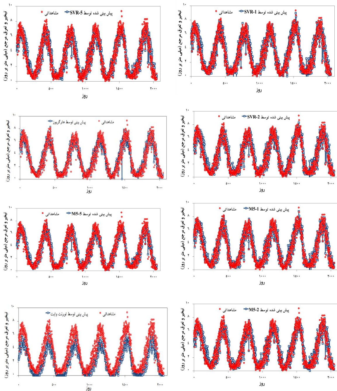
شکل ۲- نمودارهای تغییرات زمانی مقادیر تبخیر و تعرق مرجع با استفاده از روش فائو- پنمن- مونتهیث و روش‌های SVR، M5 و روش‌های تجربی تورنت وایت و هارگریوز
