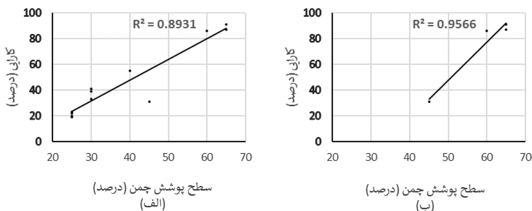
شکل ۱۴- (الف) تغییرات کارایی نوارهای حائل گیاهی حاوی چمن و درصد سطح پوشش گیاه چمن در طول دوره آزمایش (ب) تغییرات کارایی نوارهای حائل گیاهی حاوی چمن و درصد سطح پوشش گیاه چمن در چهار ماه ابتدایی آزمایش Figure14. (a) Variations of the efficiency of turf grass buffer strips and vegetation cover during the study period (b) Variations of the efficiency of turf grass buffer strips and vegetation cover during the first four months of the study
