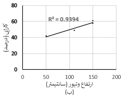
شکل ۸- الف) تغییرات کارایی نوارهای حائل گیاهی حاوی وتیور و ارتفاع گیاه وتیور در طول دوره آزمایش ب) تغییرات کارایی نوارهای حائل گیاهی حاوی وتیور و ارتفاع گیاه وتیور در چهار ماه ابتدایی آزمایش Figure 8. (a) Variations of the efficiency of vetiver buffer strips and vetiver grass height during the study period (b) Variations of the efficiency of vetiver buffer strips and vetiver grass height during the first four months of the study
