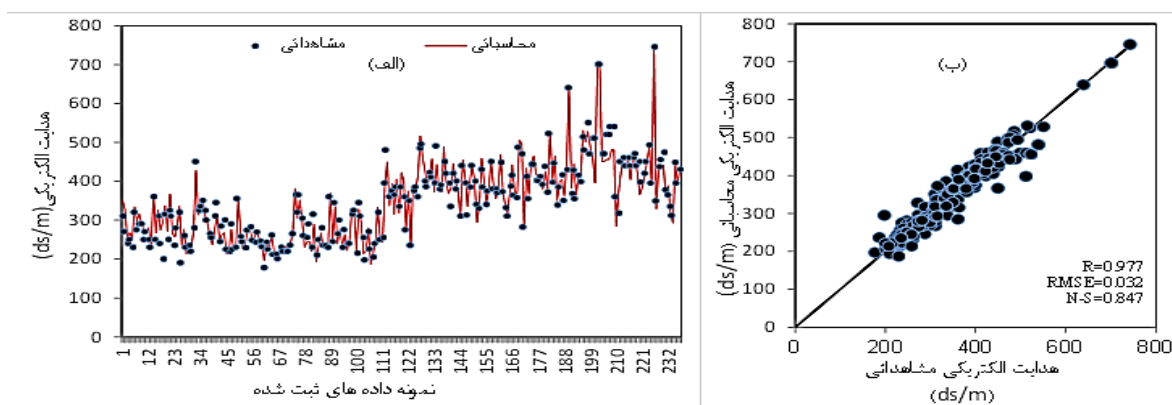
شکل ۴- نمودار حاصل از مقادیر بهینه مدل شبکه عصبی موجک برای داده‌های ثبت‌شده مرحله آموزش و صحت سنجی
