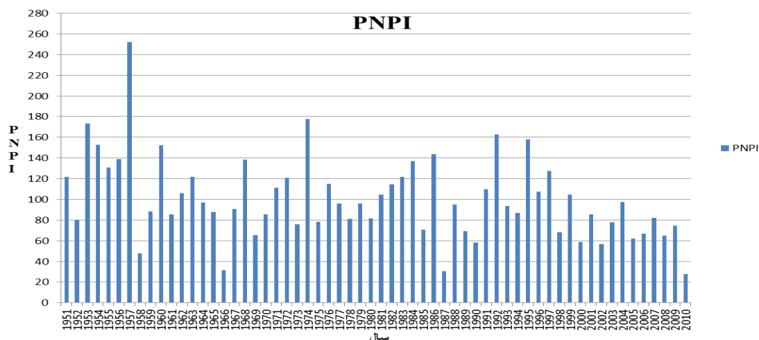
شکل ۱۱- تعیین و طبقه‌بندی ترسالی‌ها، خشکسالی‌ها و بارش‌های نرمال در استان کرمان به روش PNPI Figure 11. Determination and classification of wetlands, droughts and normal precipitations in Kerman province with PNPI method
