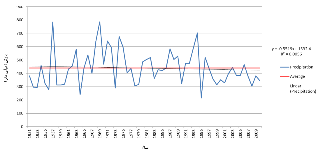
شکل ۱- تغییرات بارندگی سالانه استان کرمانشاه Figure 1. Annual precipitation changes in Kermanshah province
