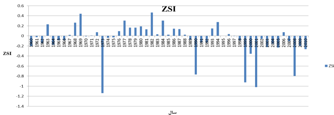
شکل ۱۴- تعیین و طبقه‌بندی ترسالی‌ها، خشکسالی‌ها و بارش‌های نرمال در استان کردستان به روش ZSI Figure 14. Determination and classification of wetlands, droughts and normal precipitations in Kordestan province with ZSI method
