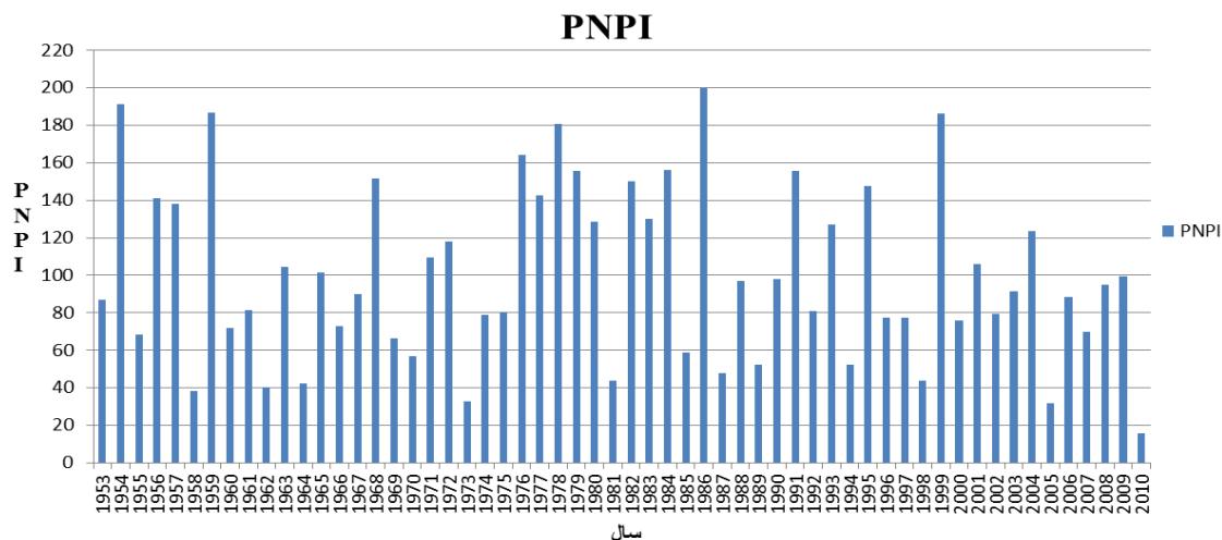
شکل ۱۲- تعیین و طبقه‌بندی ترسالی‌ها، خشکسالی‌ها و بارش‌های نرمال در استان یزد به روش PNPI Figure 12. Determination and classification of wetlands, droughts and normal precipitations in Yazd province with PNPI method
