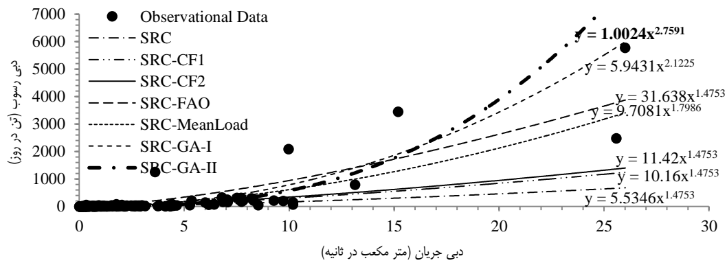
شکل ۵- برازش مدل‌های مختلف منحنی سنج رسوب به داده‌های مشاهداتی (مجموعه داده واسنجی) Figure 5. Fitness of various SRC models to the observational data (calibration data set)
