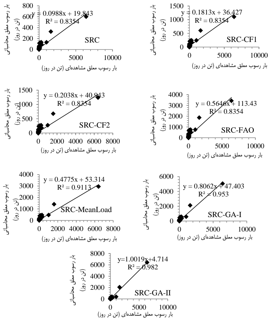
شکل ۶- نمودارهای پراکنش نقطه‌ای دبی رسوب معلق محاسباتی - مشاهده‌ای (مرحله آزمون) مدل‌های مختلف منحنی سنج رسوب Figure 6. Scatter plots of observed and estimated SSL (SSL for the test data set) from different SRC models
