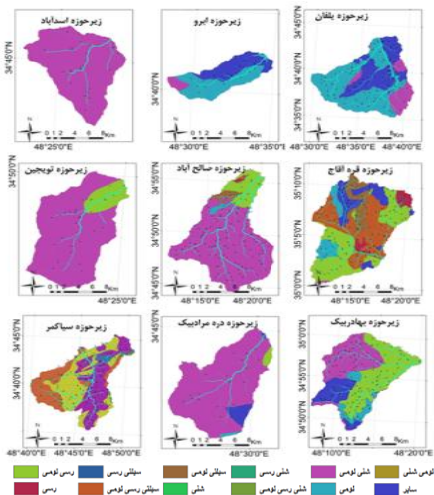
شکل ۳- نقشه ویژگی‌های تیپ خاک در زیرحوضه‌های آبخیز Figure 3. Map of soil type characteristics in the sub-basins
