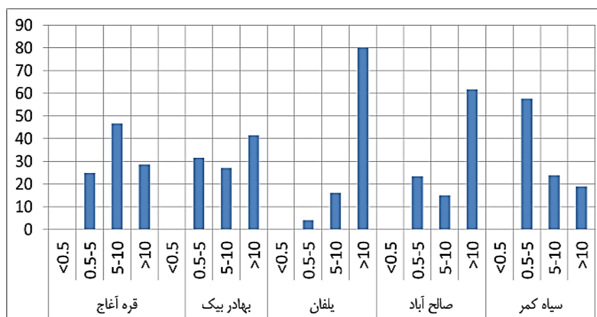
شکل ۵- درصد مساحت شیب در برخی از زیر حوضه‌ها Figure 5. The percentage of slop area in some of sub- basins
