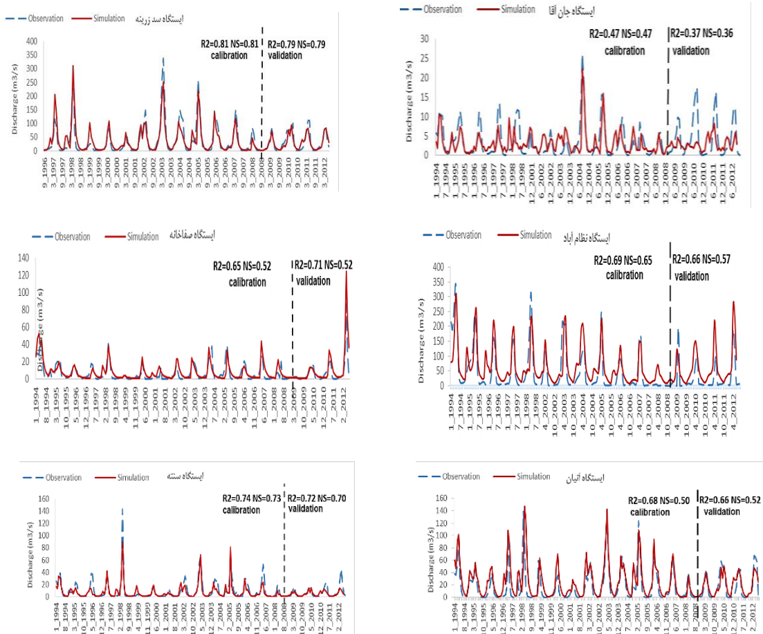
شکل ۲- نتایج واسنجی و صحت‌سنجی دبی ایستگاه‌های مختلف و نیترات کل حوزه زربینه‌رود در ماه‌های مختلف سال Figure 2. Calibration and Validation Results of Different Stations and Total Nitrate of Zarinehrood Basin
