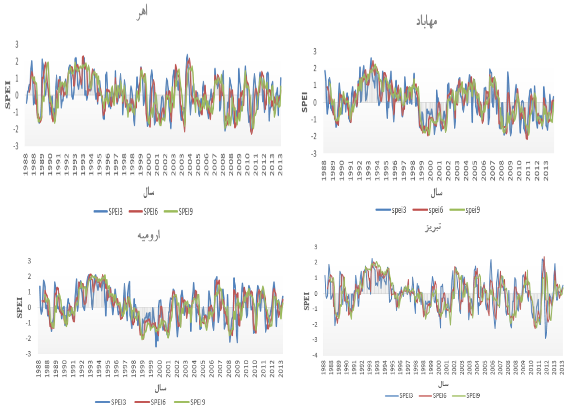
شکل ۳-مقایسه توزیع زمانی SPEI 3 ، SPEI 6 ، SPEI 9 در ایستگاههای سینوپتیک حوزه دریاچه ارومیه Figure 3. Comparison of temporal distribution of SPEI 3 , SPEI 6 , SPEI 9 in synoptic stations of Urmia Lake Basin
