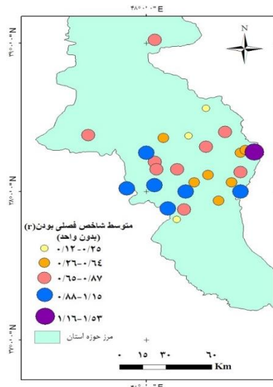
شکل ۳- نقشه مقادیر شاخص فصلی‌بودن (r) در ایستگاه‌های باران‌سنجی استان اردبیل با روش آمار دورانی Figure 3. Map of seasonality index (r) values in rain gauge stations in the Ardabil province by using circular statistical method
