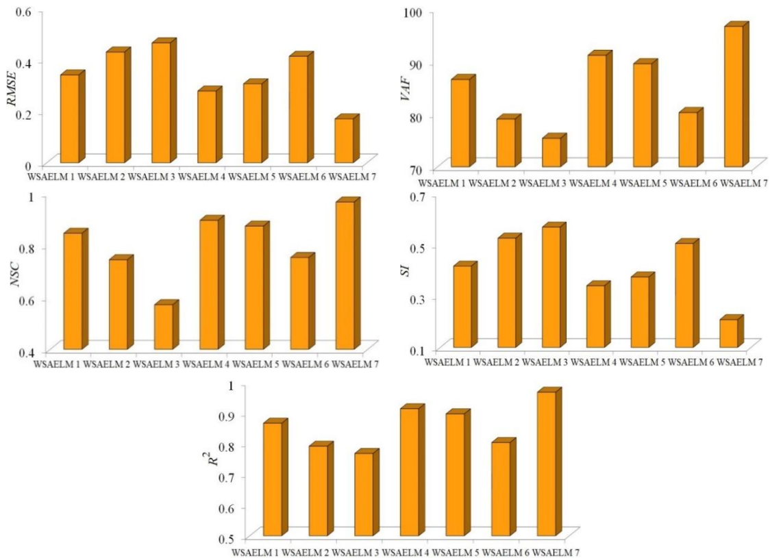
شکل ۵- نتایج شاخص‌های آماری برای شبه‌سازی توسط مدل‌های WSAELM مختلف Figure 5. Results of statistical indices for simulating rainfall values with different WSAELM models
