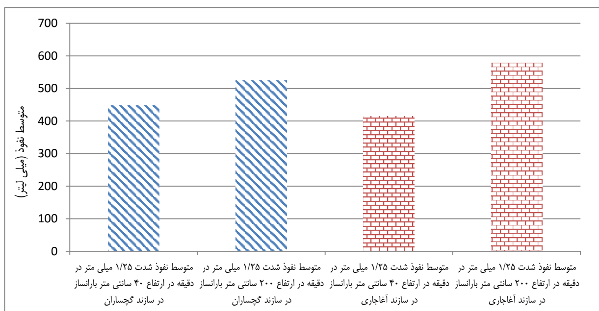
شکل ۹- مقایسه متوسط میزان نفوذپذیری در ارتفاع‌های مختلف شبیه‌ساز باران و در شدت ۱/۲۵ میلی‌متر در دقیقه در کاربری مرتع سازندهای گچساران و آغاجاری
