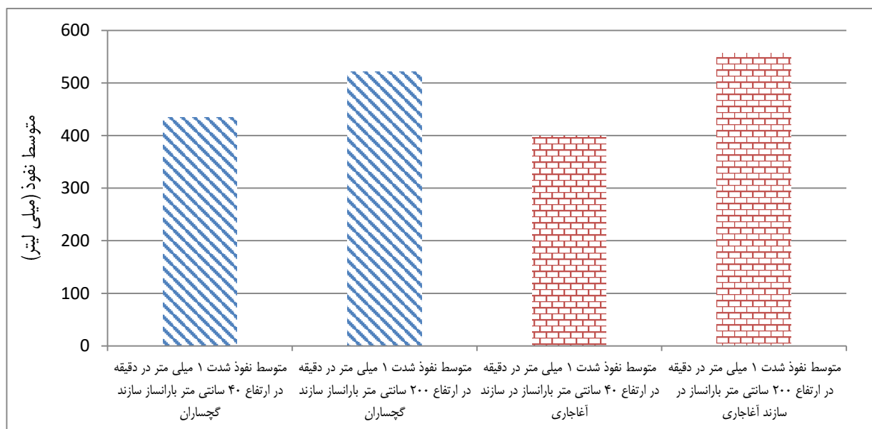
شکل ۸- مقایسه متوسط میزان نفوذپذیری در ارتفاع‌های مختلف شبیه‌ساز باران و در شدت ۱ میلی‌متر در دقیقه در کاربری مرتع سازندهای گچساران و آغاجاری
