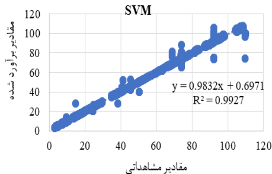
شکل ۳- مقادیر پیش‌بینی و مشاهده‌ای سطح آب زیرزمینی با مدل ماشین بردار پشتیبان (SVM)
