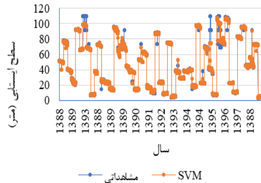
شکل ۳- مقادیر پیش‌بینی و مشاهده‌ای سطح آب زیرزمینی با مدل ماشین بردار پشتیبان (SVM)
