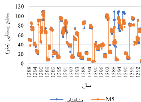
شکل ۴- مقادیر پیش‌بینی و مشاهده‌ای سطح آب زیرزمینی با مدل درخت تصمیم (M5)
