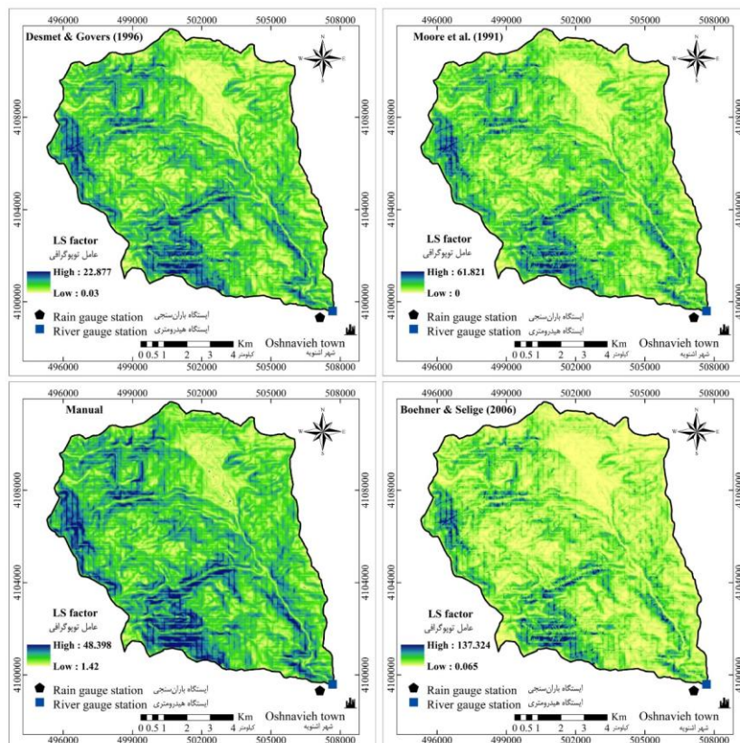
شکل ۳- نقشه عامل توپوگرافی (LS) حاصل از روش‌های محاسباتی (Desmet and Govers (1996)، Moore et al. (1991)، Boehner and Selige (2006) و روش دستی حوزه آبخیز گلازچای، استان آذربایجان غربی
