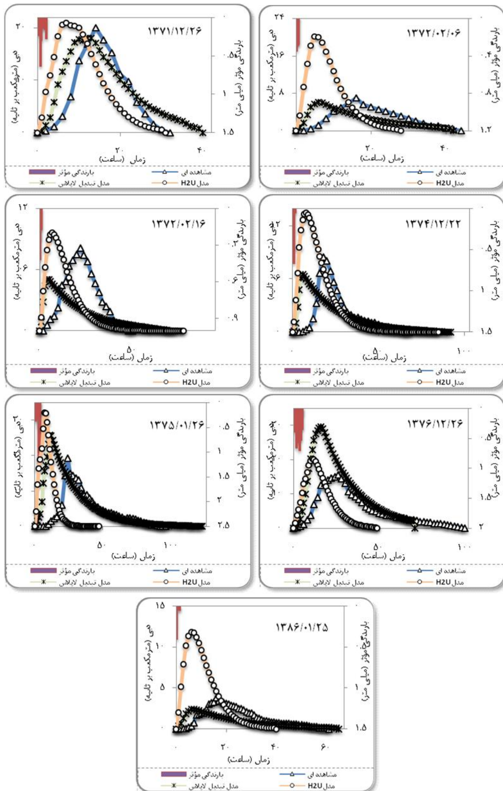
شکل ۲- آنمودهای شبیه‌سازی شده و مشاهده‌ای.
