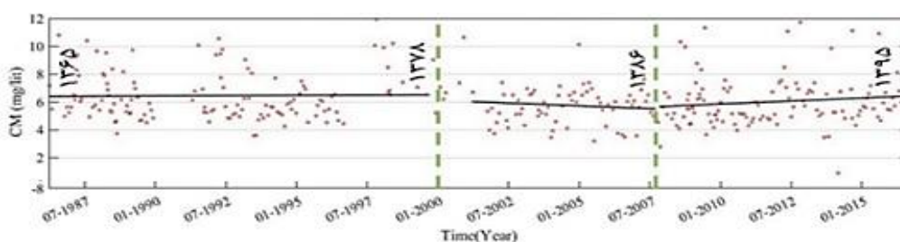
شکل ۷- تعیین سال شروع تغییر در روند بار معلق در طول دوره آماری مورد مطالعه در ایستگاه رسوب‌سنجی تمر
