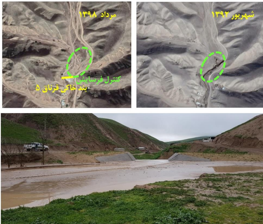
شکل ۴- بند خاکی قرناق ۵ احداث شده در سال ۱۳۹۷ Figure 4. Gheragh5 Earth dam constructed in 2018
