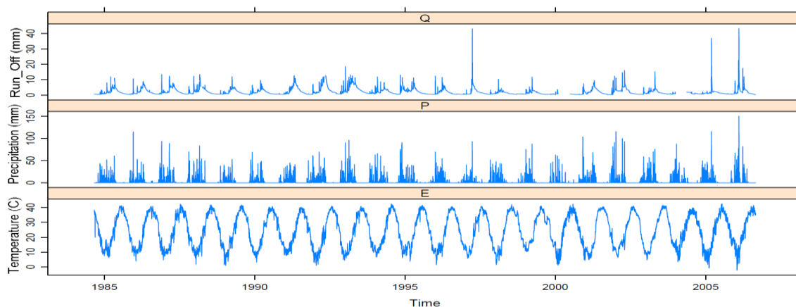
شکل ۳- سری زمانی داده‌های مشاهده‌ای ارتفاع رواناب، بارش و دما در منطقه مورد مطالعه
