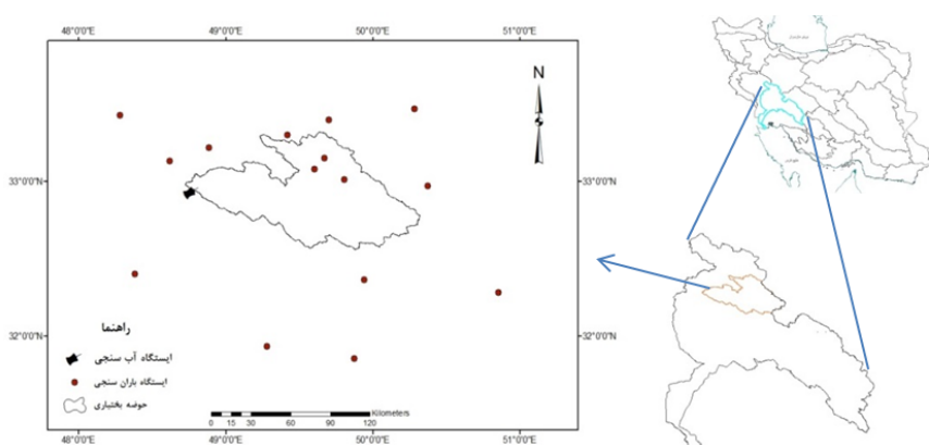
شکل ۱- موقعیت منطقه مورد مطالعه در ایران و حوضه کارون بزرگ Figure 1. Bakhtiari watershed location in Iran and Karoon catchment
