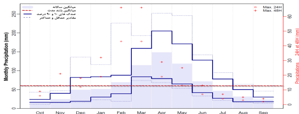
شکل ۲- رژیم ماهانه بارش در منطقه مورد مطالعه (۱۹۸۴-۲۰۰۶)
