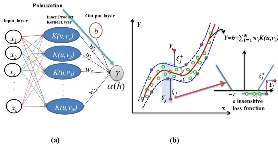
شکل ۴- نمونه‌ای از معماری ماشین بردار گرگسیونی Figure 4. An example of regression vector machine architecture
